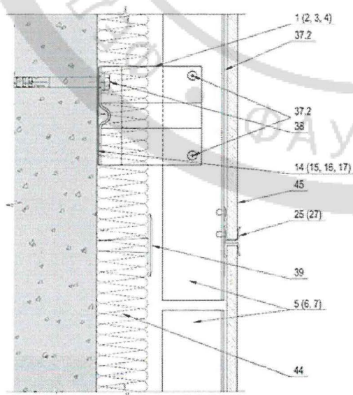
Рис.1. НФС с облицовкой керамогранитными плитами
