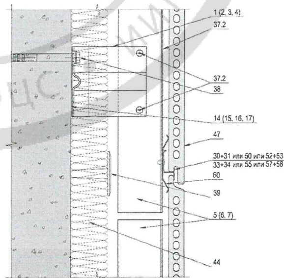
Рис.2. НФС с облицовкой керамическими плитами
